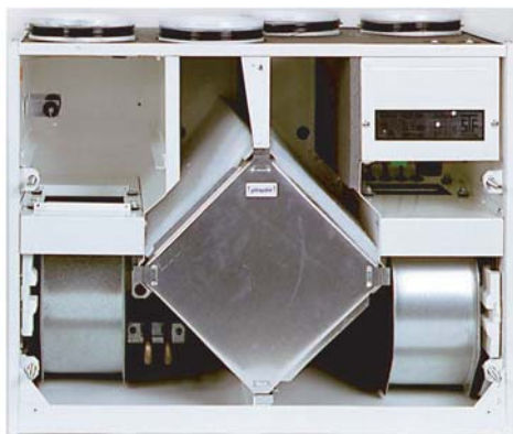
Вид без передней панели ILTO 260
