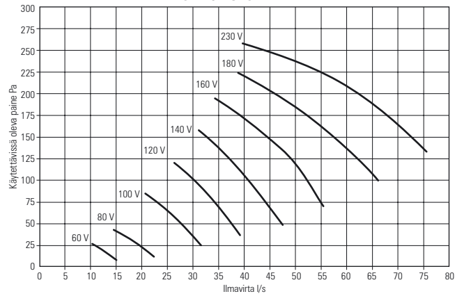
ILTO 270 TULOILMAVIRTA
