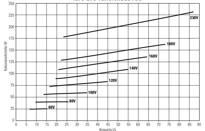
ILTO 270 TEHONKULUTUS
