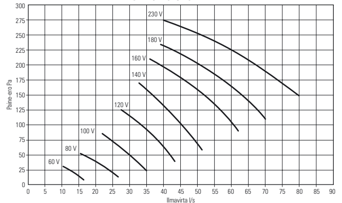
ILTO 270 POISTOILMAVIRTA
